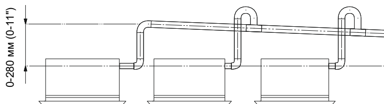
Т-образное соединение дренажных труб
