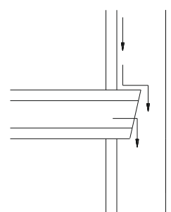
Горизонтальное соединение
