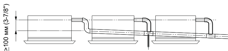
Т-образное соединение дренажных труб
